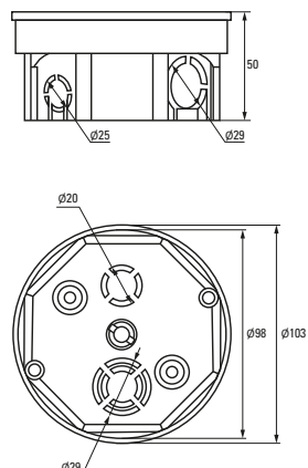
Коробка установочная KMT-010-005
