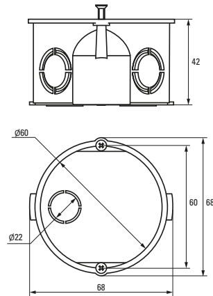
Коробка установочная KMT-010-003
