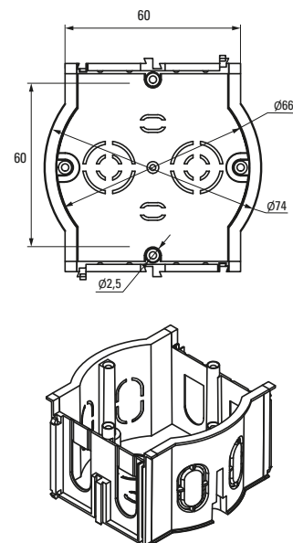
Коробка установочная КМТ-010-4007
