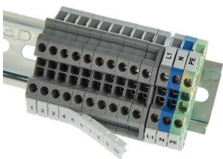
Возможна групповая маркировка клемм
