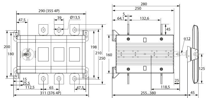
Ревёрсивный рубильник 630-800 A
