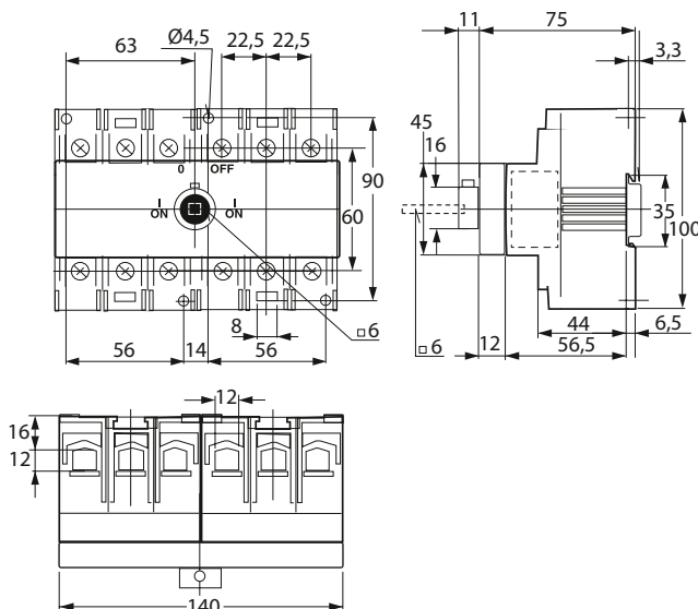
Ревёрсивный рубильник 40-125 A
