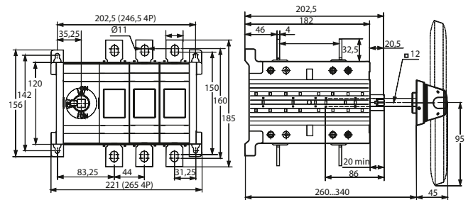
Ревёрсивный рубильник 630-800 A
