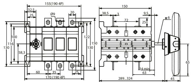
Ревёрсивный рубильник 315-400 A
