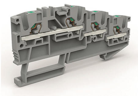
Внешний вид
