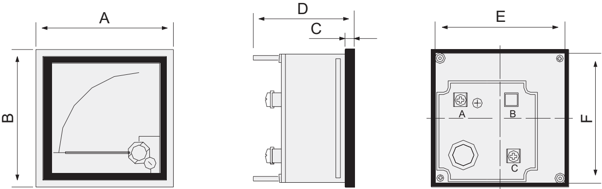
Габаритные и установочные размеры, мм
