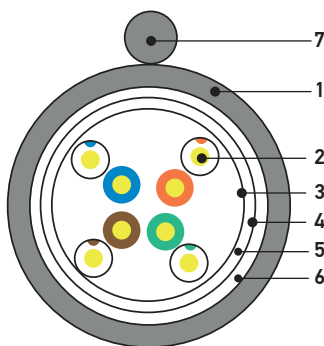
Конструкция кабеля F/UTP с тросом
