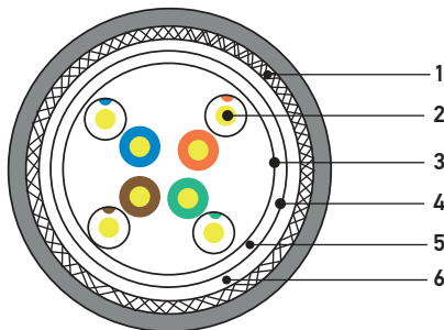
Конструкция кабеля SF/UTP
