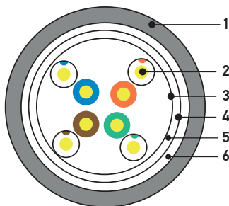
Конструкция кабеля F/UTP
