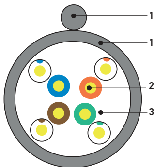
Конструкция кабеля U/UTP с тросом
