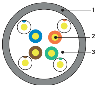
Конструкция кабеля U/UTP
