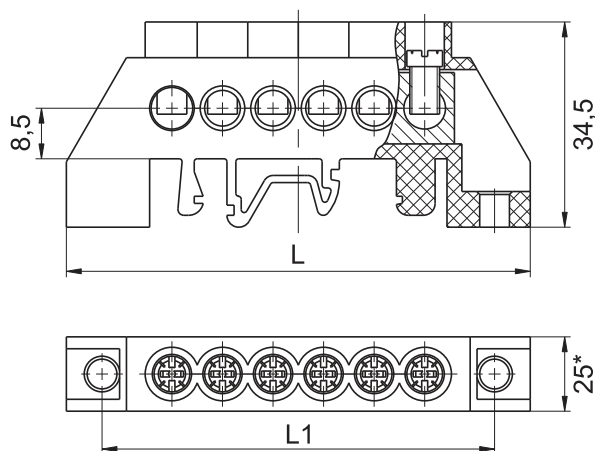
Рисунок 5 – Шина РЕ «земля» (N «ноль», L «фаза») в корпусном изоляторе на DIN-рейку
