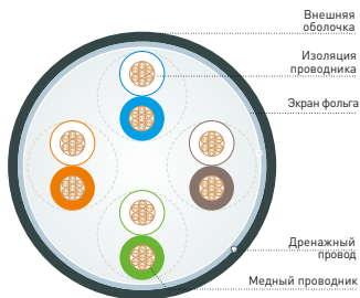
Рис. 2 – Конструкция патч-корда категории 5E типа F/UTP
