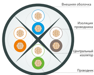
Рис. 3 – Конструкция патч-корда категории 6 типа U/UTP
