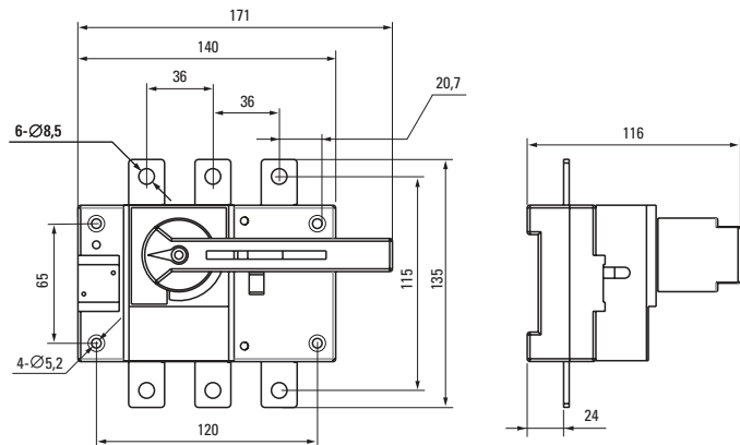
Рисунок 1а – Монтажные размеры рубильника PowerSwitch 160 A трехполюсного
