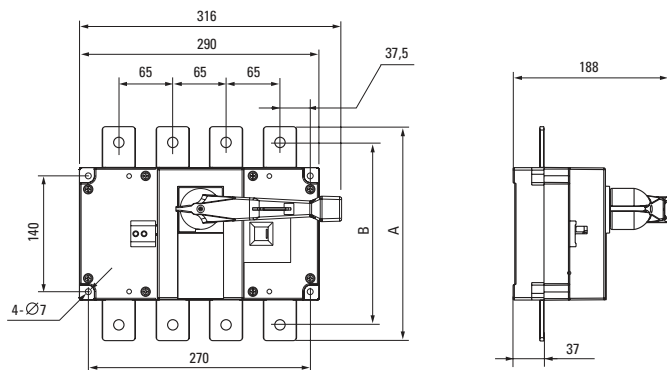
Рисунок 36 – Монтажные размеры рубильника PowerSwitch 400-630 A четырехполюсного
