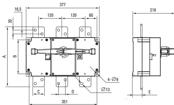
Рисунок 4а – Монтажные размеры рубильника PowerSwitch 1000-1600 A трехполюсного
