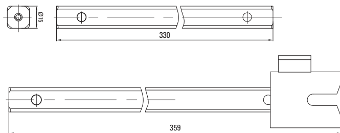
Рисунок 7б – габаритные чертежи штока ( 800~3150А)
