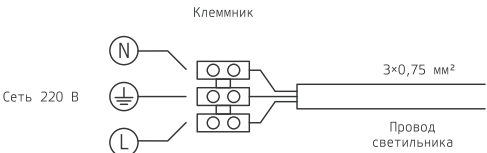
Рис. 1. Схема подключения светодиодного светильника к сети 220 В
