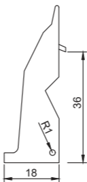
Рис. 9 - Габаритные размеры держателя PM-22-36 EKF AVERES
