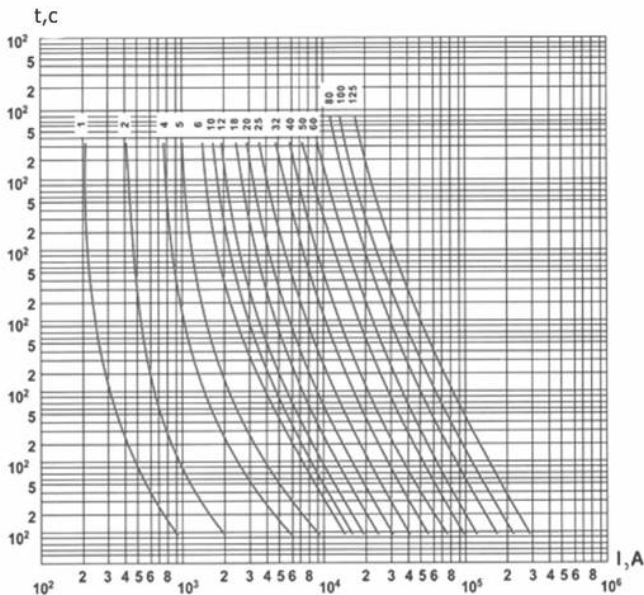
Рис. 2 Времятоковые характеристики ПВЦ
