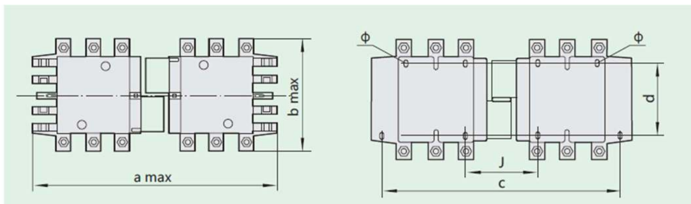
Рисунок 2 Габаритные и установочные размеры контакторов переменного тока серии NC2-115Ns~800Ns
