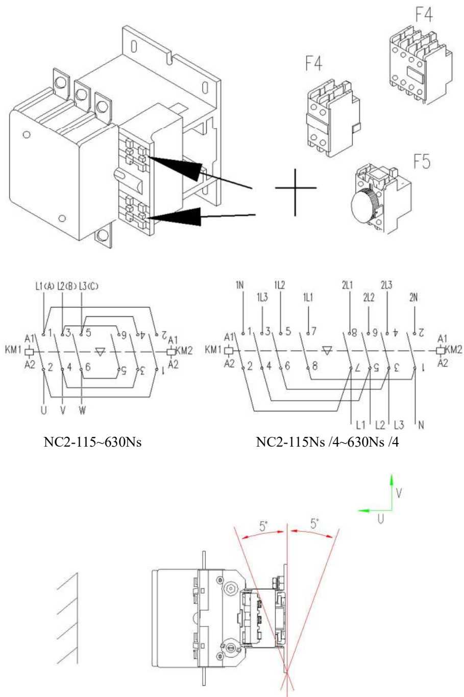
Условия монтажа
