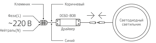
Рис. 2. Схема подключения светодиодного светильника к электросети 220 В
