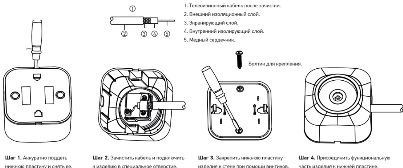
Рисунок 3. Схема сборки телевизионной розетки серии FREA (ТОКОВ™).
